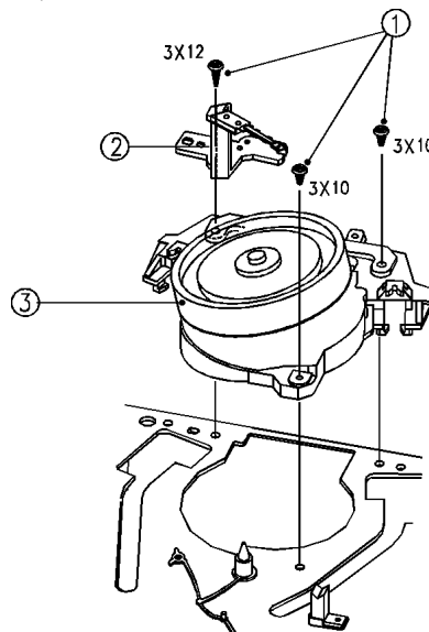
Drum total assembly and earth bracket assembly removal. Entfernen von walzenbausatz & erdklemmbausatz.
