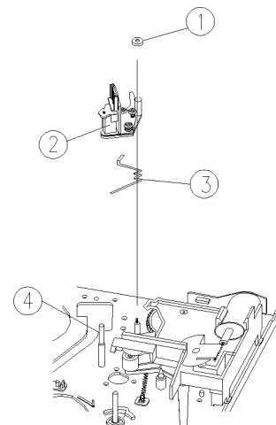
Disassembly of the AC head assembly Zerlegen des audio-steuerkopf-bausatzes
