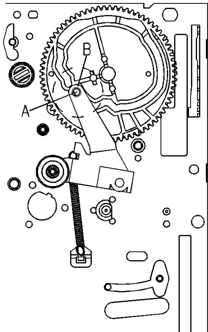
Datum position of pinch lever total assembly and cam gear Bezugsposition von abschnürhebel-gesamtbausatz & nockensteuerung
