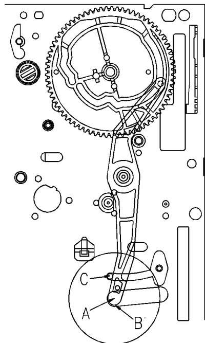
Datum position of relay lever Bezugsposition vonrelais-hebel & nockengsteuerung
