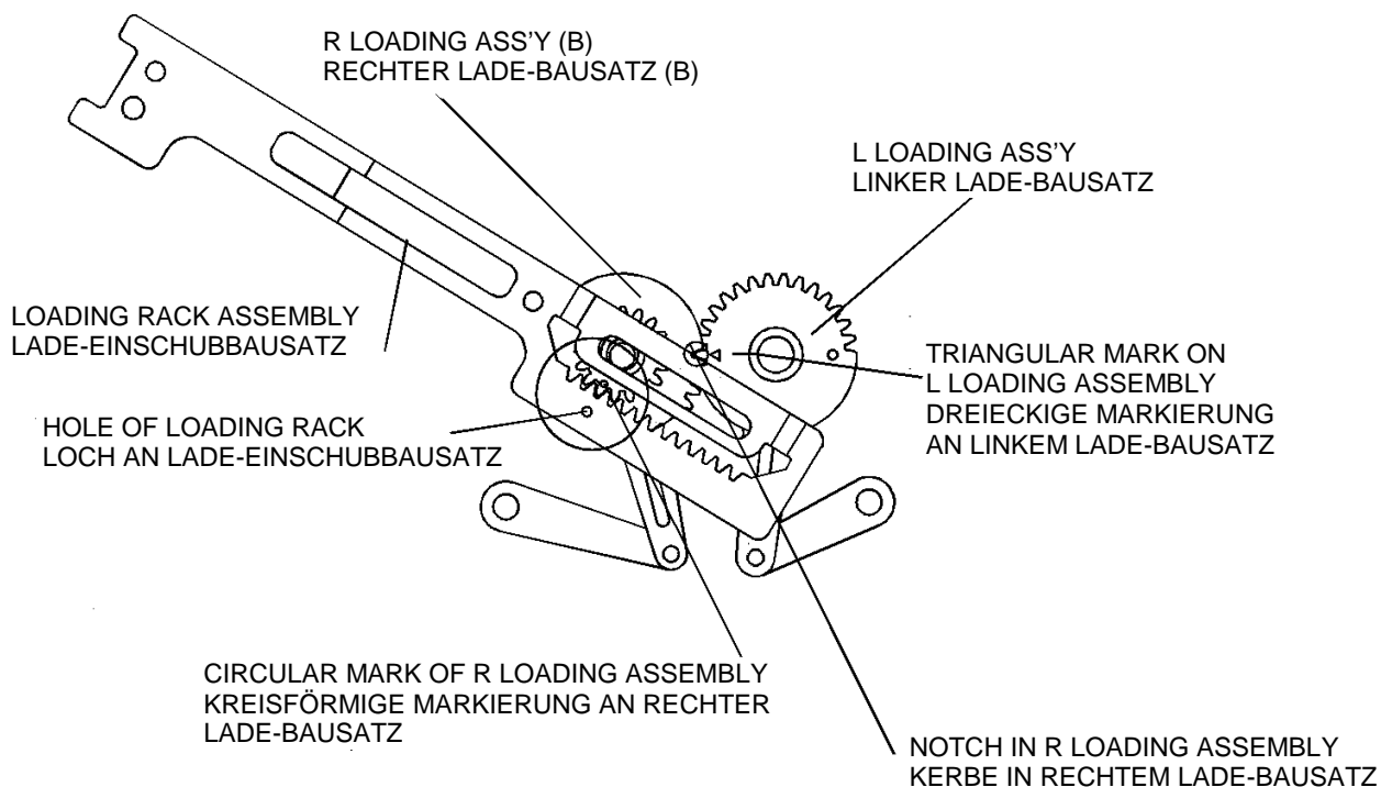
Datum position of loading rack assembly and R/L loading lever assemblies Bezugsposition von lade-einschubbausatz & r / ladehebel-bausatz
