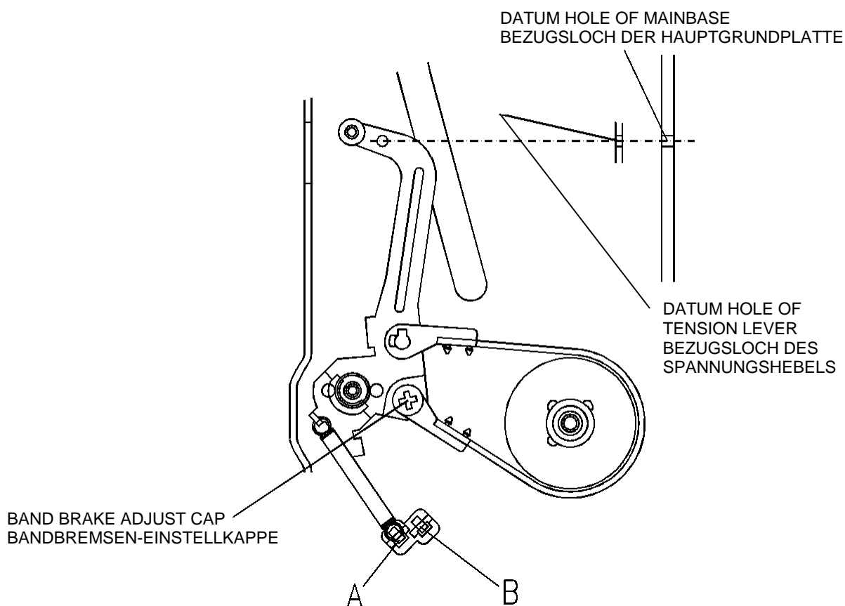
Tension pole position adjustment Einstellung der spannungspolposition
