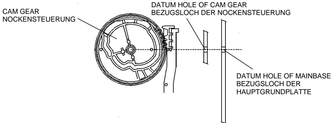
Datum position of F/L rack and cam gear Bezugsposition von F/L-einschub & nockengsteuerung
