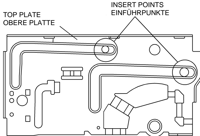
Assembly of the F/L Assembly Zusammenbau des F/L-Bausatzes
