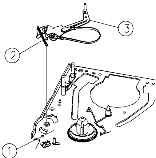
Tension band assembly removal Entfernen des spannungsband-bausatzes
