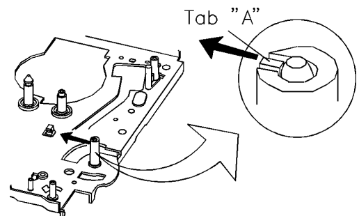
Tension band assembly removal Entfernen des spannungsband-bausatzes
