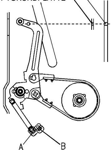
Adjustment of the tension pole position Einstellung der spannungspolposition
