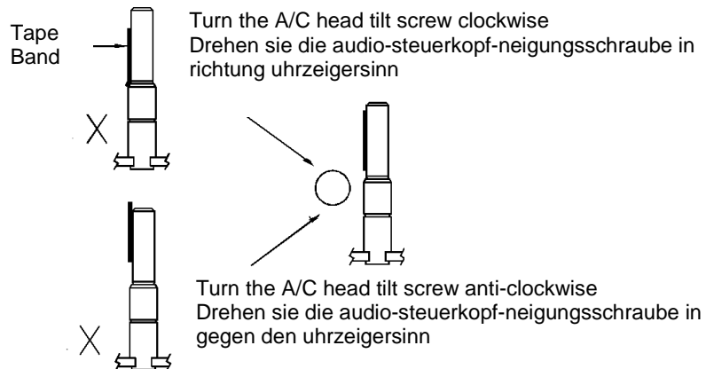
A/C head assembly adjustment Neigungseinstellung des audio-steuerkopf-bausatzes
