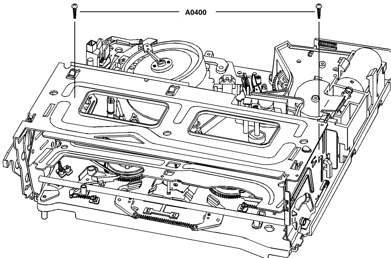
Front loading assembly separation Entfernen des frontladebausatzes
