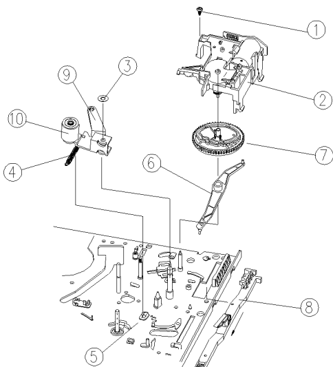
L/C bracket, pinch lever, cam gear, relay lever, F/L rack removal Entfernen von H/N-Klammer, abschnurhebel, nockensteuerung, relais-hebel, F/L-einschub
